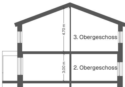
Schnitt (1:200 - DIN A4)
